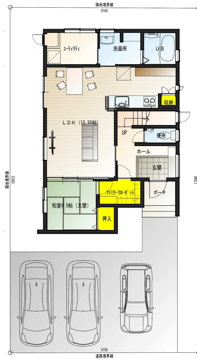
1階平面図
